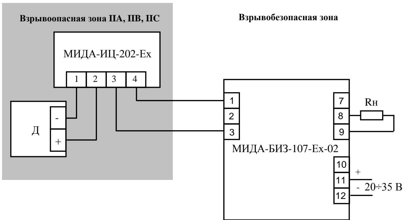
Рисунок Г.2 – Схема подключения индикатора с барьером искрозащиты измерительным МИИД-БИЗ-107-Ех
